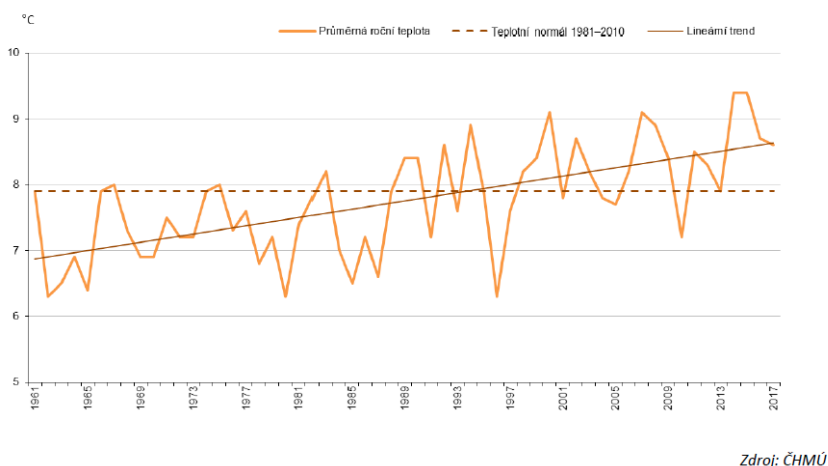
Dlouhodobý vývoj průměrné roční teploty vzduchu na území ČR ve srovnání s normálem 1981–2010, 1961–2017 [°C]
